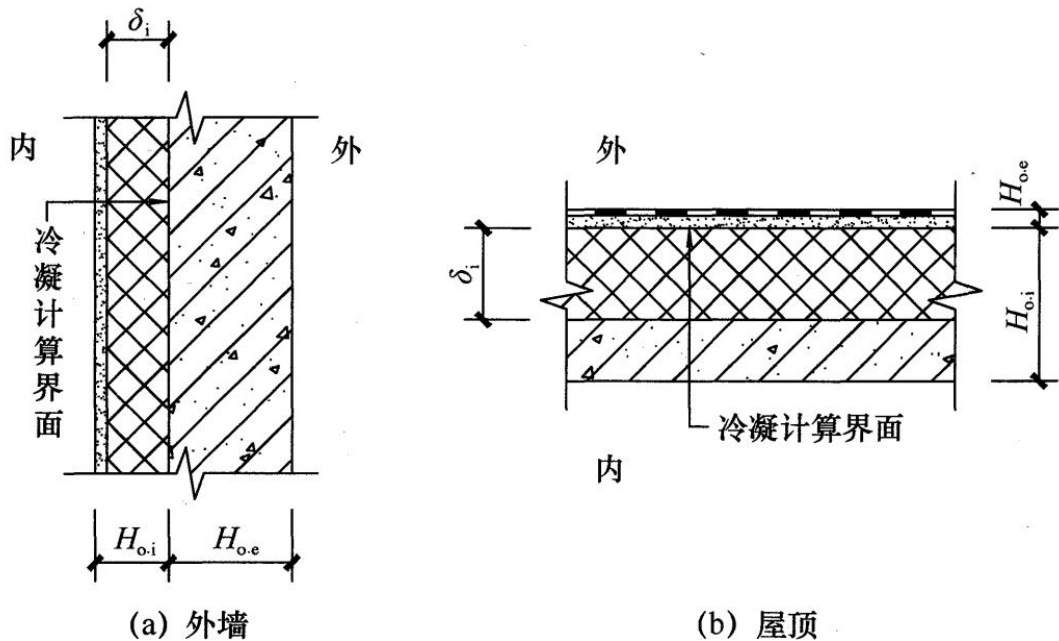
图 7.1.6 冷凝计算界面
